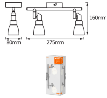
Technische Daten Ledvance LED-Spot G9 Aluminium 2x 4W - 827 Extra Warmweiß
